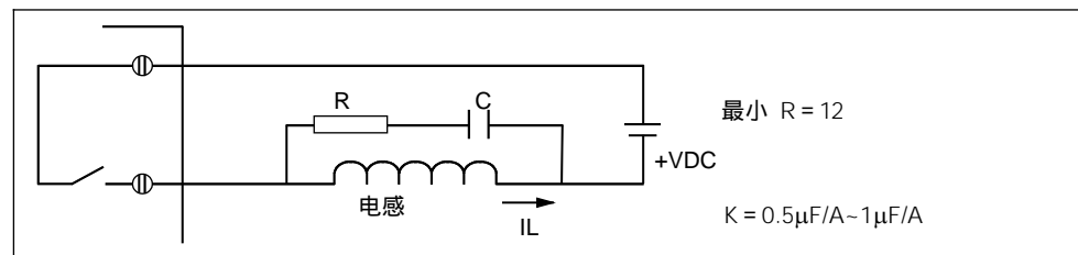
图 47 继电器驱动 DC 负载上跨接电阻电容网络保护电路
