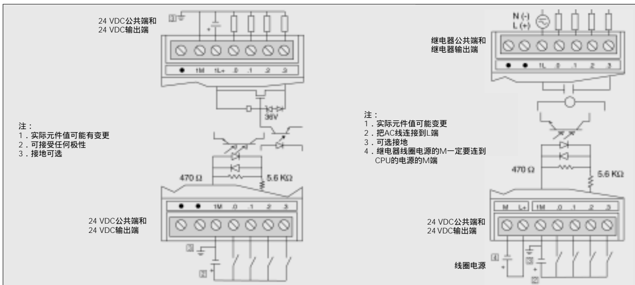
图 24 EM 223 4 × 24V DC 输入/4 × 24V DC、继电器输出端子连接图 ( 6ES7 223-1BF22-0XA0、6ES7 223-1HF22-0XA0 )
