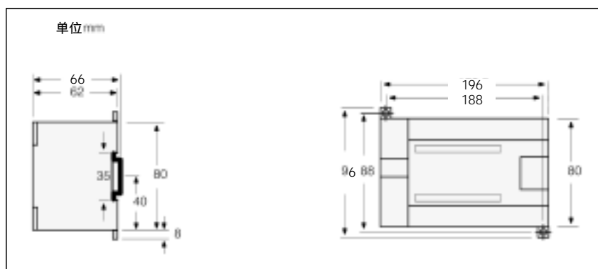
图 16 CPU226 尺寸图
