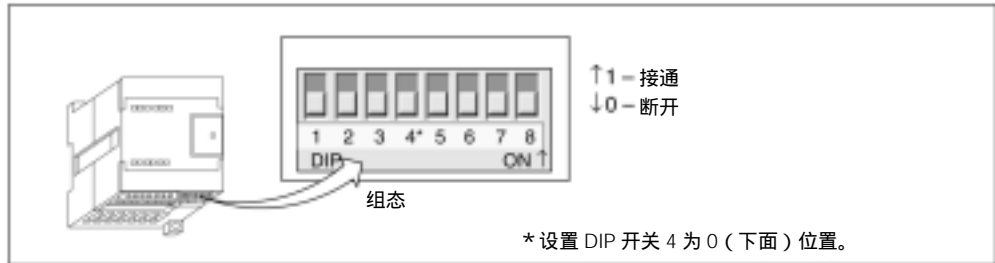
图 32 组态热电阻模块的 DIP 开关。
