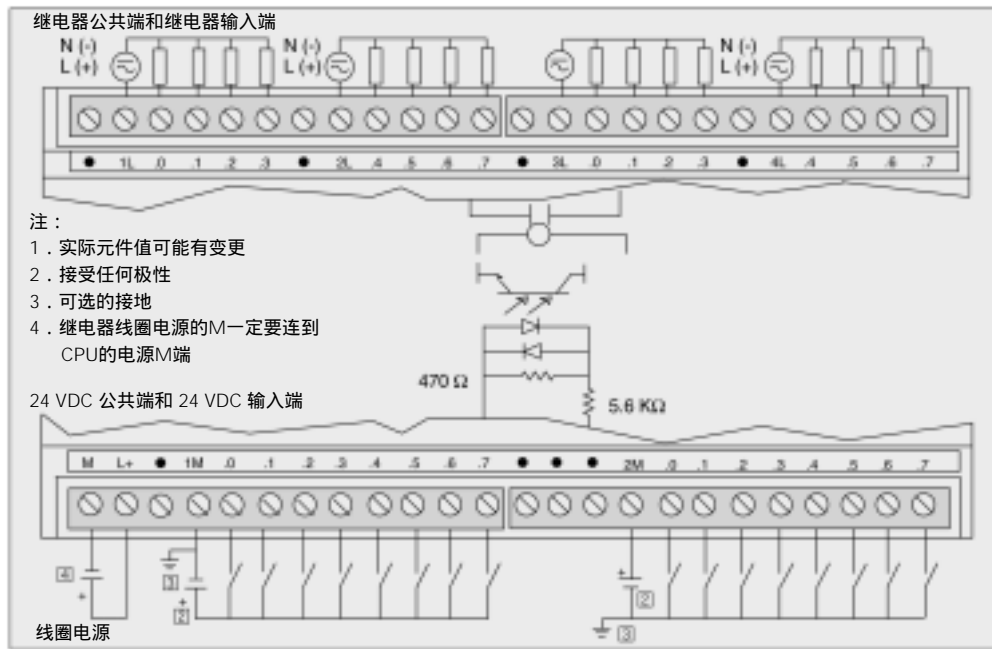
图 27 EM 223 16 × 24V DC 输入/16X 继电器输出端子连接图 (6ES7 223-1PL22-0XA0)
