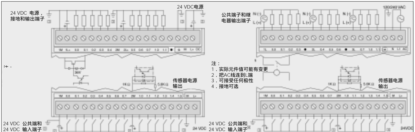
图 10 CPU224 端子连接图 (6ES7 214-1AD23-0XB0、6ES7 214-1BD23-0XB0)
