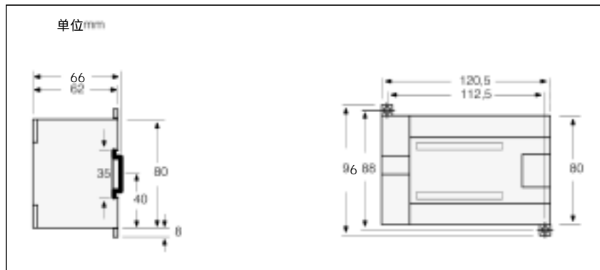
图 15 CPU224 尺寸图
