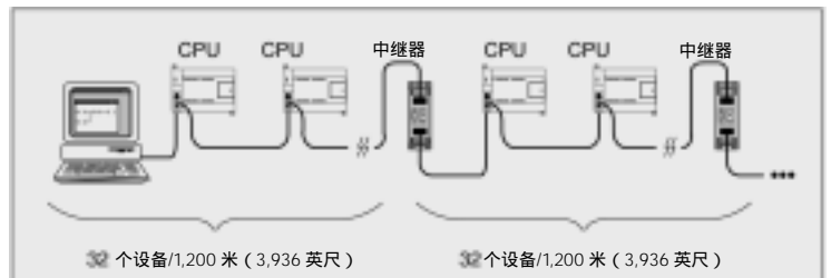
图 2 带有中继器的网络
