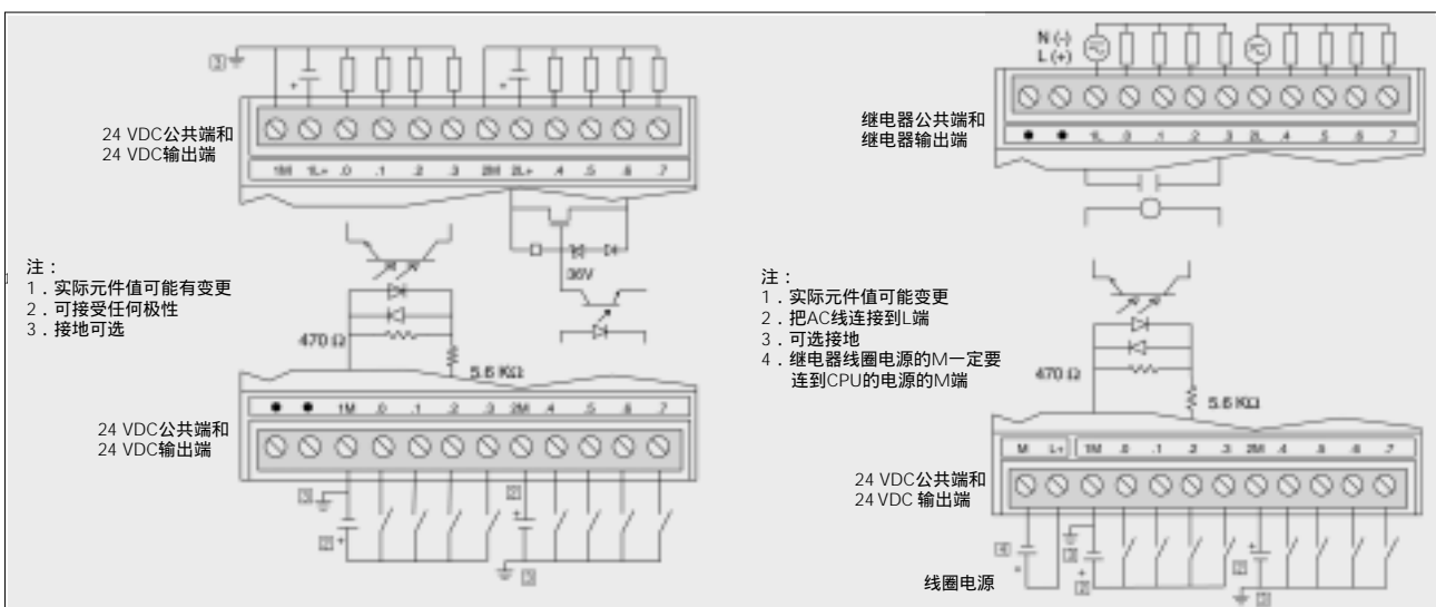
图 25 EM 223 8 × 24V DC 输入/8 × 24V DC、继电器输出连接端子图 ( 6ES7 223-1BH22-0XA0、6ES7 223-1PH22-0XA0 )
