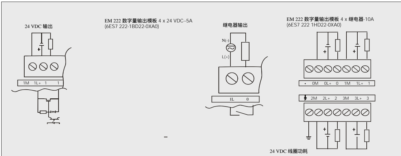
图 23 EM 222 数字量输出模板 4 × 24VDC-5A、4 × 继电器-10A ( 6ES7 222-1BD22-0XA0、6ES7 222-1HD22-0XA0 )
