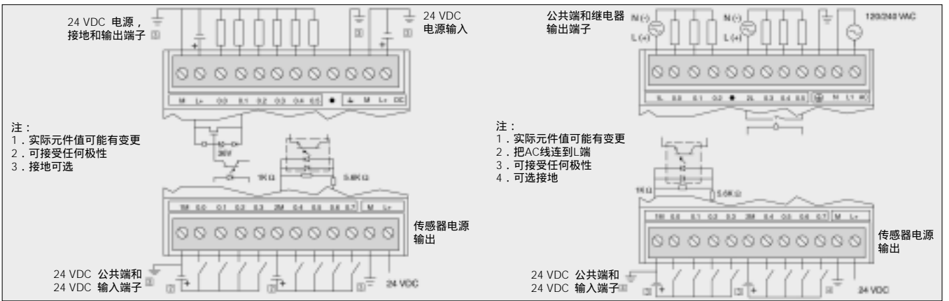
图 9 CPU222 端子连接图 (6ES7 212-1AB23-0XB0、6ES7 212-1BB23-0XB0)
